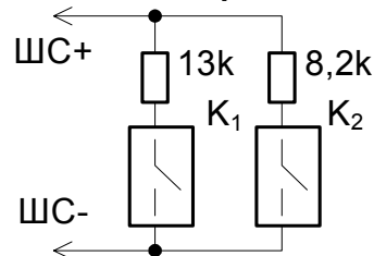
Тип 5 (охранный с контролем блокировки)
