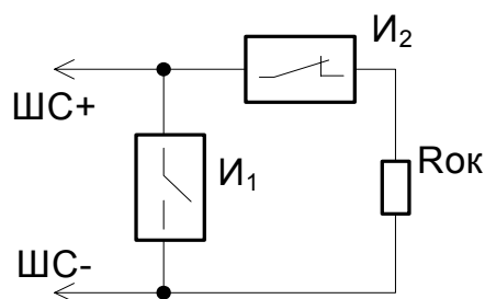
Тип 4 (охранный ШС)
