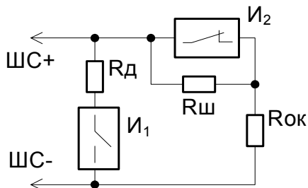
Тип 2 (пожарный комбинированный ШС)
