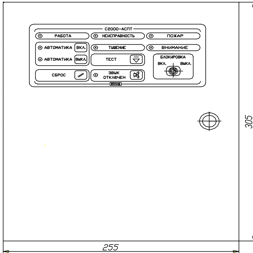
Установочные размеры
