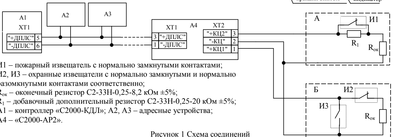
Рисунок 1 Схема соединений
